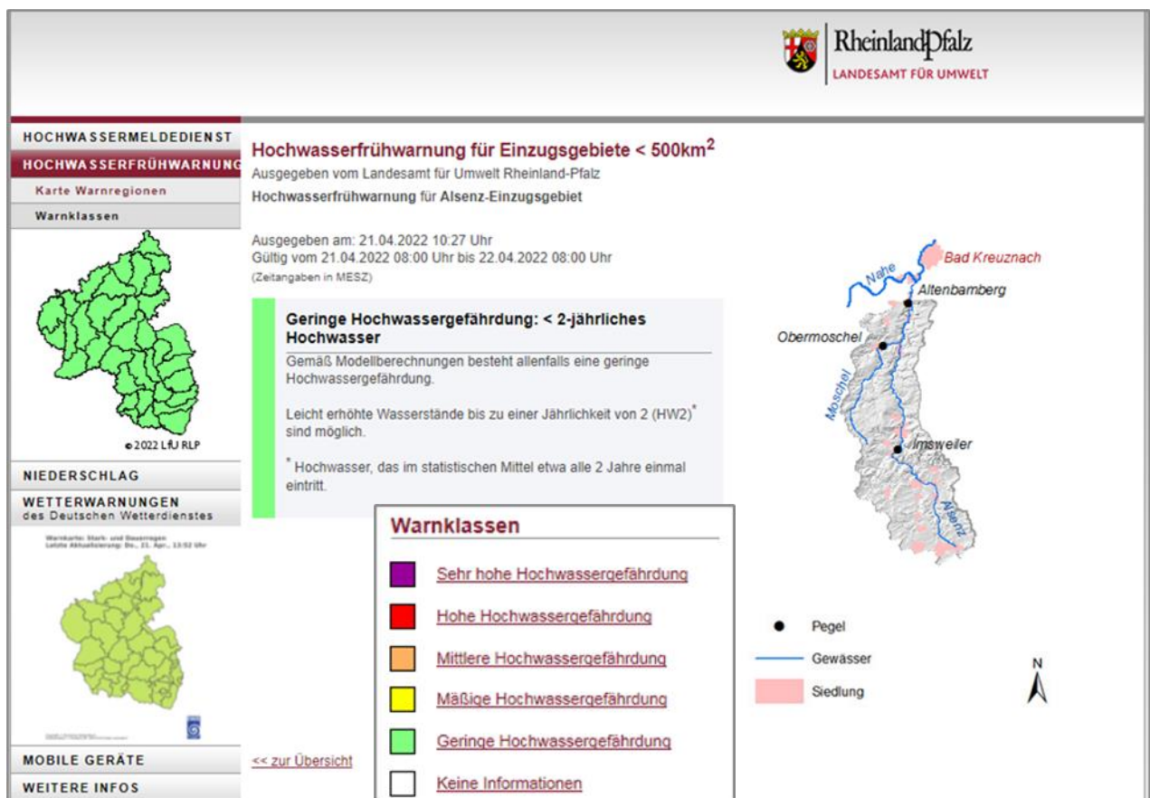
Abb. 4: Karte der Hochwasserfrühwarnung für EZG < 500 km² http://fruehwarnung.hochwasser-rlp.de/
